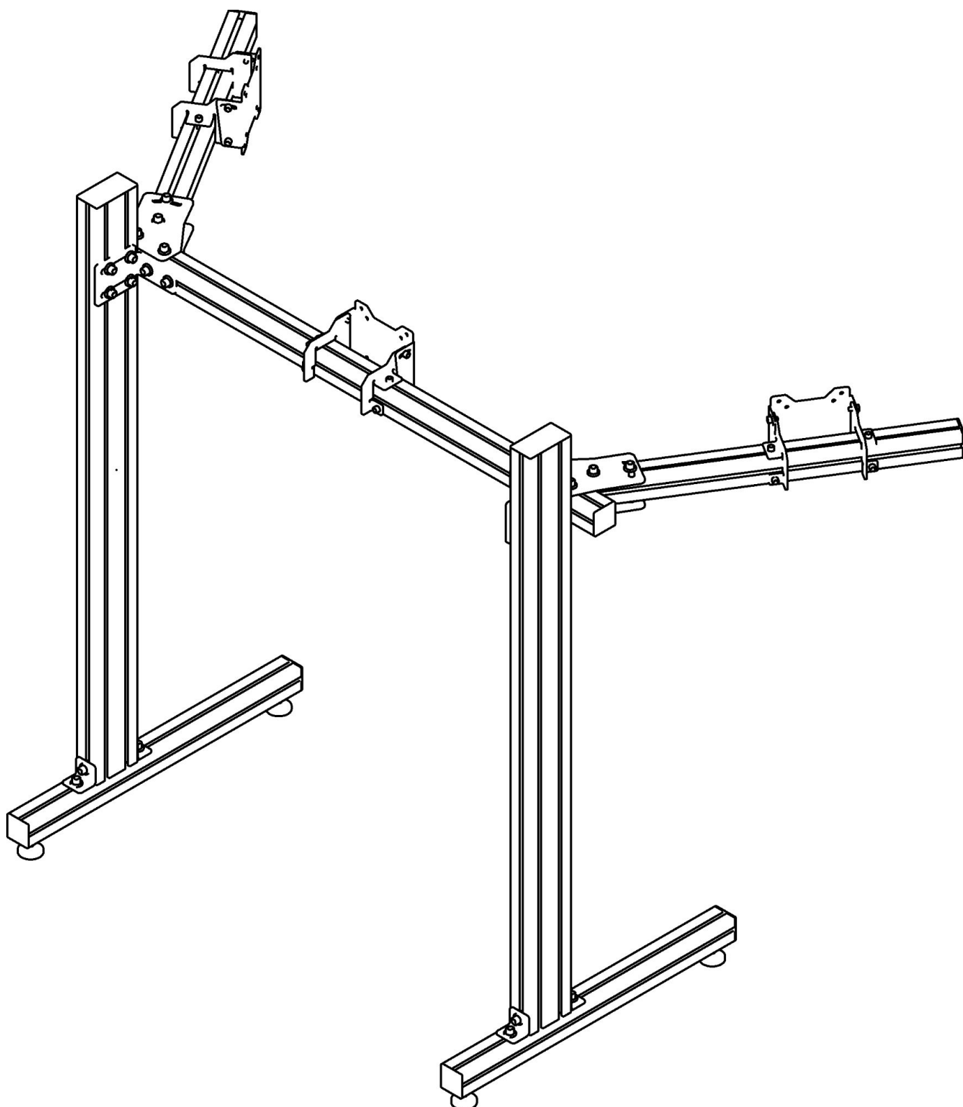
SUPORE EXTERNO PRS PRO PARA 3 MONITORES
